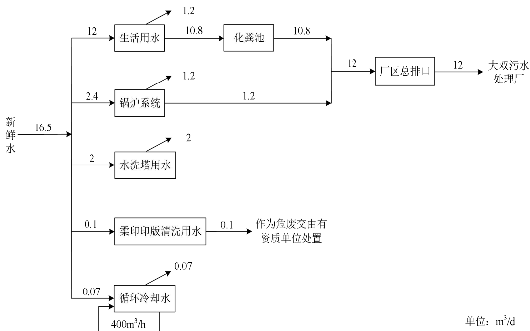
图 3.2-1 本项目水平衡图
