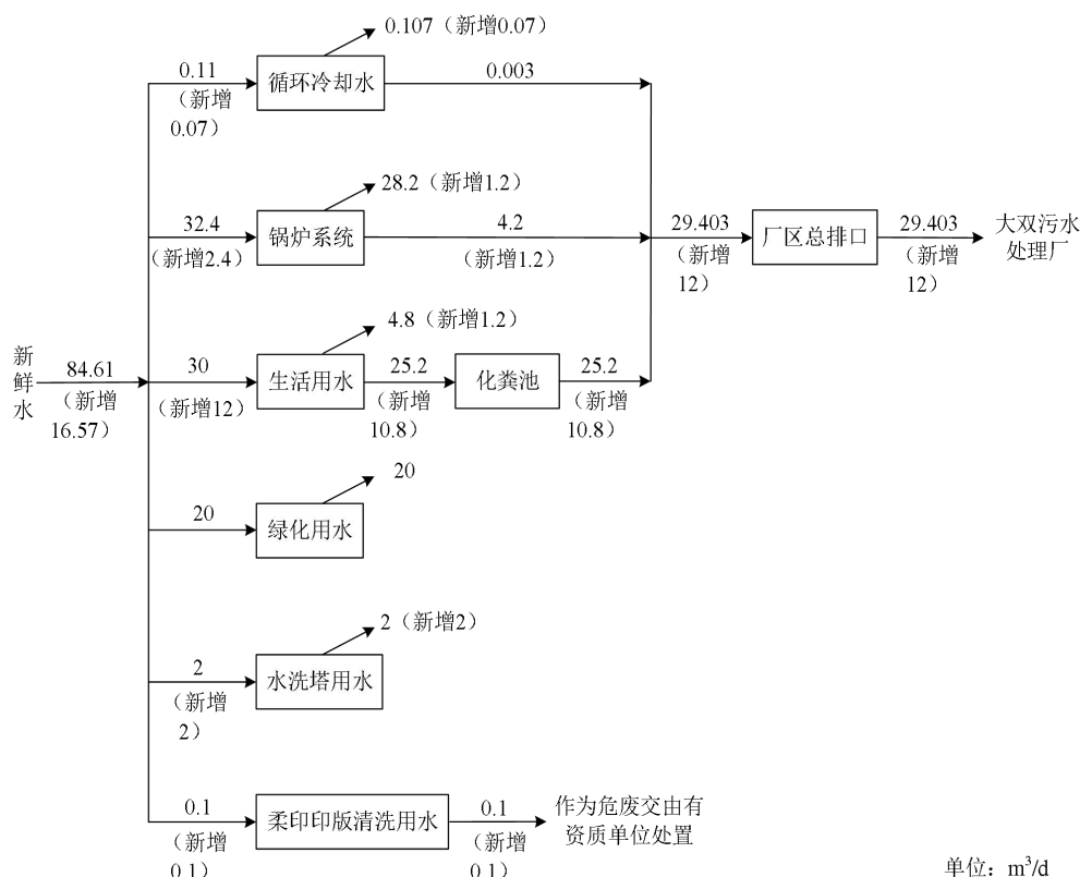
图 3.2-2 本项目实施后全厂水平衡图
