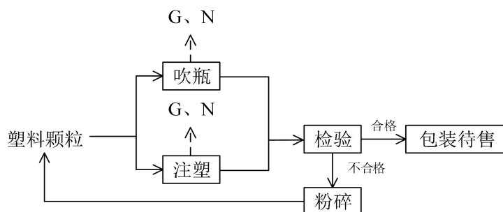
图 2.3-4 塑料瓶生产工艺流程及产排污节点示意图
