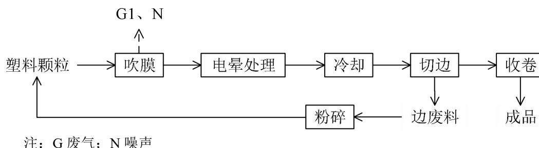
图 3.3-1 吹膜薄膜生产工艺流程图
