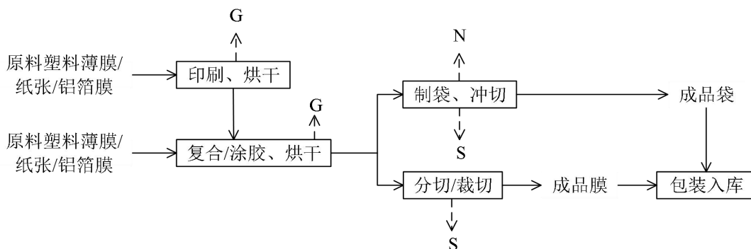
图 2.3-6 纸、铝、塑料包装材料生产工艺流程及产排污节点示意图
