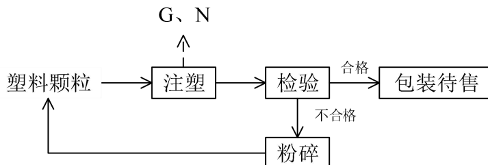
图 2.3-2 塑料杯生产工艺流程及产排污节点示意图（一）
