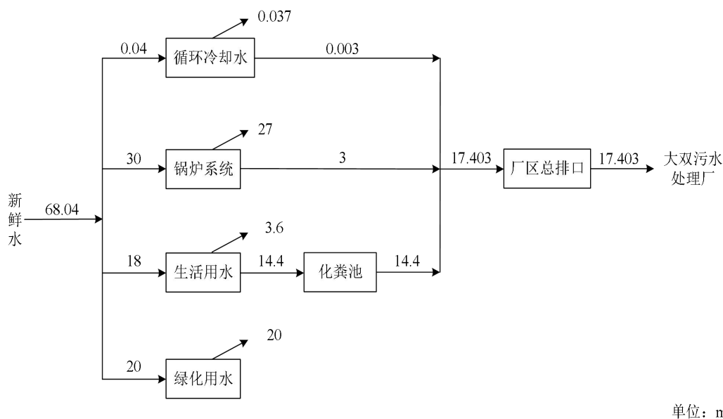
图 2.4-1 现有工程水平衡图
