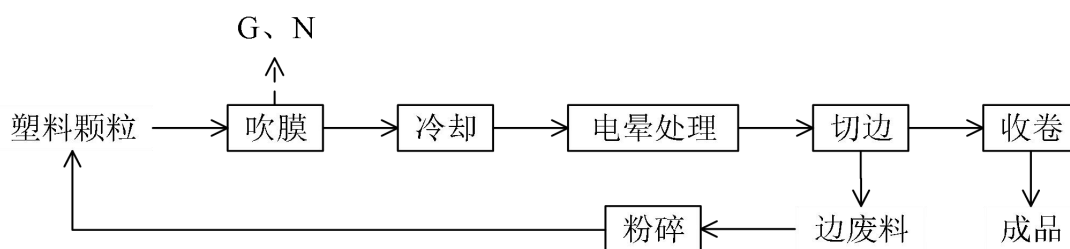
图 2.3-5 吹膜薄膜生产工艺流程及产排污节点示意图
