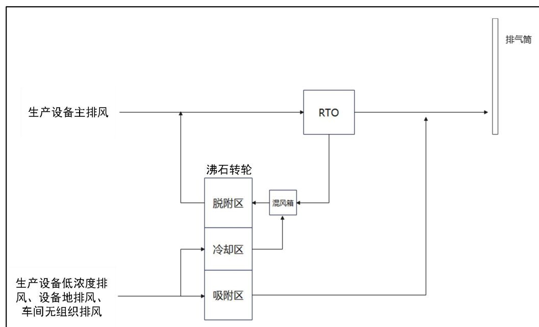
图 7.2-1 “沸石转轮+RTO”处理流程图
