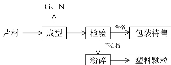
图 2.3-3 塑料杯生产工艺流程及产排污节点示意图（二）
