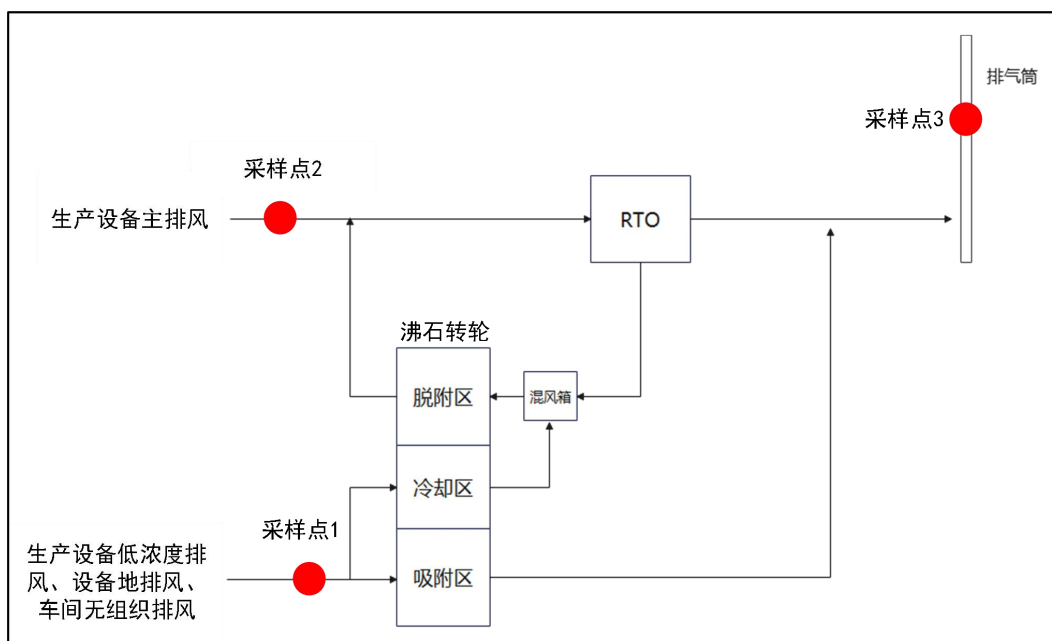
图 7.2-2 “沸石转轮+RTO” 采样点示意图
